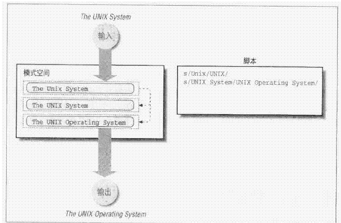
图 4-1: 脚本中的命令改变了模式模式空间的内容
